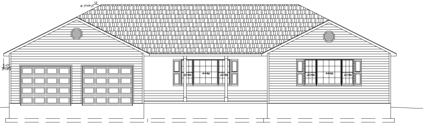
1 FRONT ELEVATION A-1 SCALE: 1/4"=1'-0"
